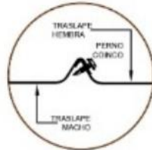
DETALLE DE FIJACIÓN
